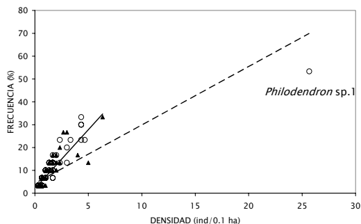
Figura 3. Distribución espacial de la abundancia de lianas y hemiepífitas en E.B. Paujil (círculos) y la C.N. Buenos Aires (triángulos). La línea de tendencia intermitente pertenece a la E.B. Paujil ( y = 2.5571x + 4.3108 , R^2 = 0.6829 , P = 6.63E-24 ), mientras que la continua pertenece a la C.N. Buenos Aires ( y = 5.1531x + 2.052 , R^2 = 0.7883 , P = 1.82E-16 ). Los valores de frecuencia están basados en el porcentaje de subunidades (2 x 50 m) en los que la especie fue registrada. Se indica la posición de la hemiepífita Philodendron sp.1 perteneciente a la E.B. Paujil.
