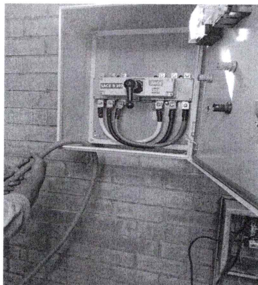
Cambio de llave de Transferencia de Grupo electrógeno
