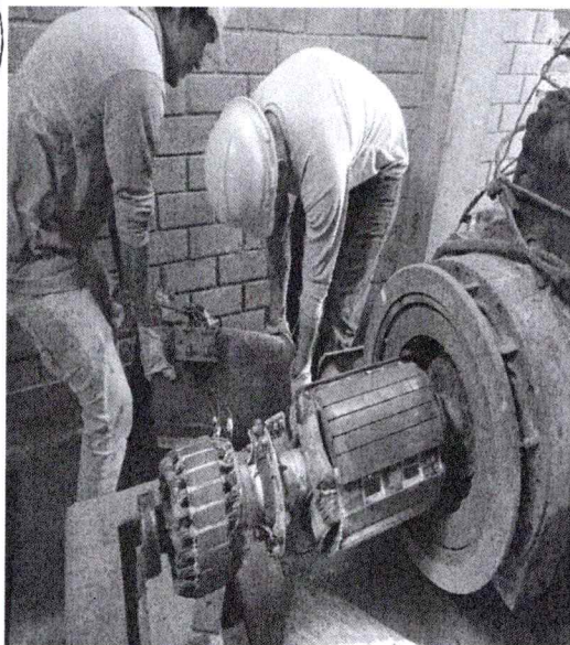
Grupo electrógeno Mantenimiento completo
